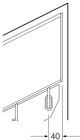
Spannstab – Ø 6 mm
