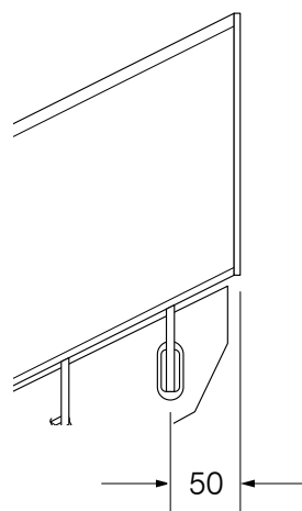
Spannseil – Ø 3,5 mm
