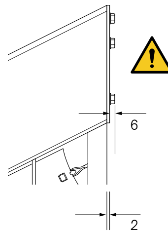
Freitragende Ausführung Achtung: Schrauben stehen über!
