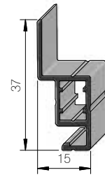
Spannrahmenprofil
