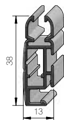
Flügelprofil
