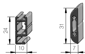
Spannrahmenprofil
