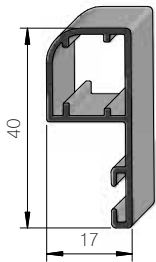
Montagerahmenprofil
