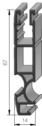
Griffprofil für SA
