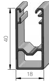
Führungsschiene
