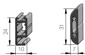
Spannrahmenprofil
