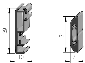
Spannrahmenprofil Sprossenprofil, nicht gewebeteilend (ab 1500 mm Höhe bzw. Breite Standard)
