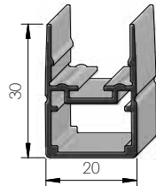
Rahmenprofil
