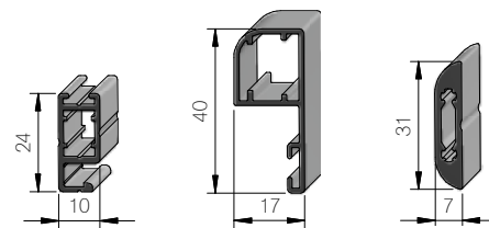
Spannrahmenprofil
