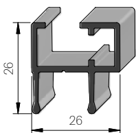
Zweifach-Führungsschiene
