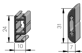
Spannrahmenprofil Sprossenprofil, nicht gewebeteilend (ab 1500 mm Höhe bzw. Breite Standard)
