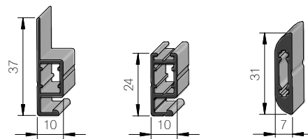
Spannrahmenprofil
