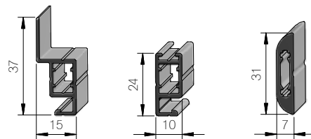
Spannrahmenprofil
