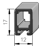
Einbaurahmenprofil
