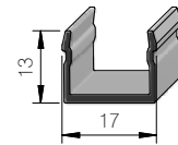
Gewebeprofil (hoch)
