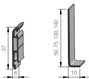
Lichtschachtprofil
