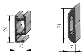
Spannrahmenprofil Sprossenprofil, nicht gewebetteilend (ab 1500 mm Höhe bzw. Breite Standard)
