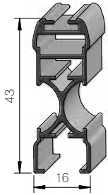
Griffprofil
