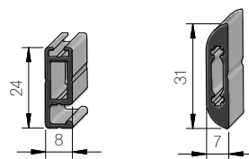
Spannrahmenprofil Sprossenprofil, nicht gewebetteilend (ab 1200 mm Höhe bzw. Breite Standard)
