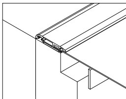
Abb. 2: Lichtschacht an Kautschukbänder befestigen
