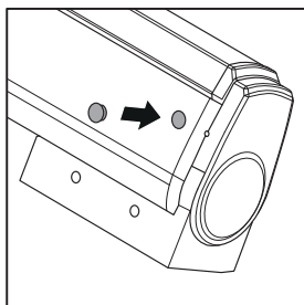
Abb. 7: Abdeckkappe wieder aufsetzen
