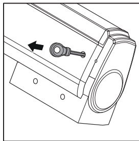
Abb. 6: Nach der Notbedienung kann die Öse, wenn gewünscht, wieder nach unten herausgezogen werden. Dabei wird der Klipp beschädigt und muss für die nächste Bedienung ausgetauscht werden.
