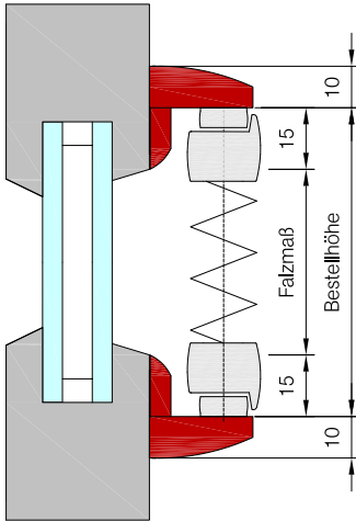
Glasleistenträger D3S (Bestellhöhe=Falzmaß-6 mm)
