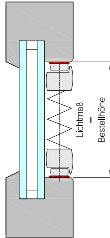
Klebträger KT 1 (Bestellhöhe=Falzmaß-8 mm)
