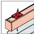
Deckenwinkel für Oberschiene XL
