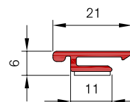
C-Profil mit Klebestreifen
