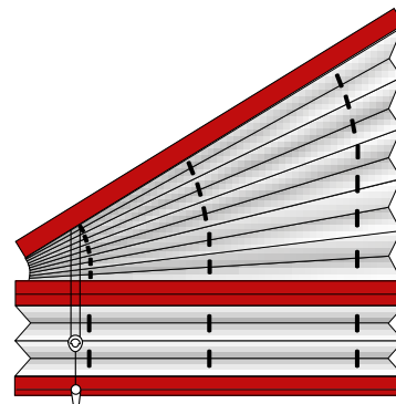
Plisseo®-Bedienung mit Schnurzug auf der niederen Seite
