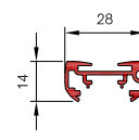
Unterschiene 28x14 mm
