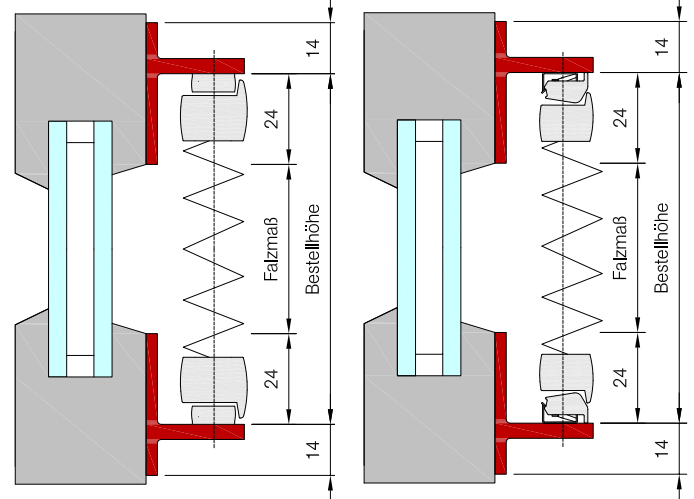
Klebträger KT 2 / Klebträger KT 3 (Bestellhöhe=Falzmaß+48 mm)
